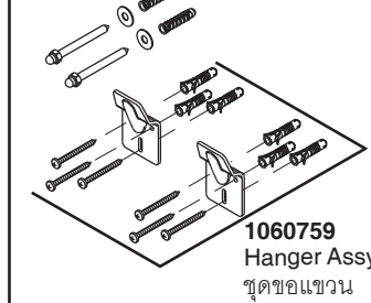
1206734 Hanger Assy ขอแขวน
