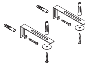
1017138 Accessory Kit ชุดอุปกรณ์ยึดอ่างล้างหน้า
