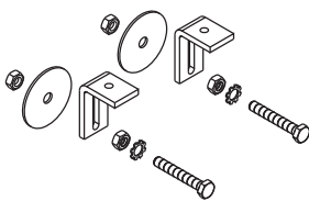
1017137 Accessory Kit ชุดอุปกรณ์ยึดอ่างล้างหน้า
